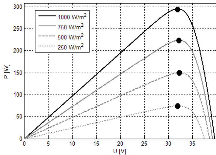
Rys. 4. Wpływ zmiany natężenia promieniowania słonecznego na wydajność modułu fotowoltaicznego Fig. 4. Effect of change in solar radiation intensity on photovoltaic module efficiency
