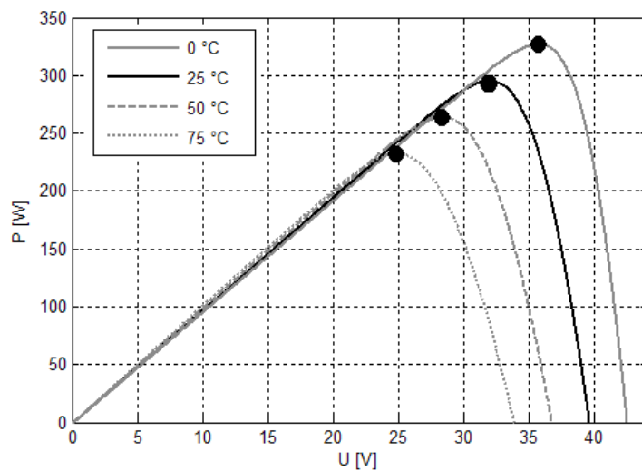
Rys. 5. Wpływ zmiany temperatury pracy modułu fotowoltaicznego na jego wydajność Fig. 5. Effect of changes of the photovoltaic module operating temperature on its performance
