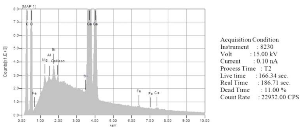
Rys. 5. Widmo pierwiastkowe w pierwszym mikroobszarze próbki G6
